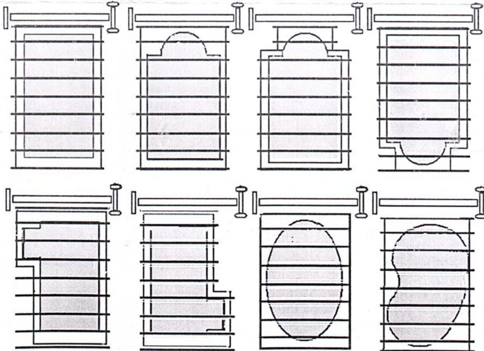
Formes fréquentes et possibilités de situation de l'enrouleur.
